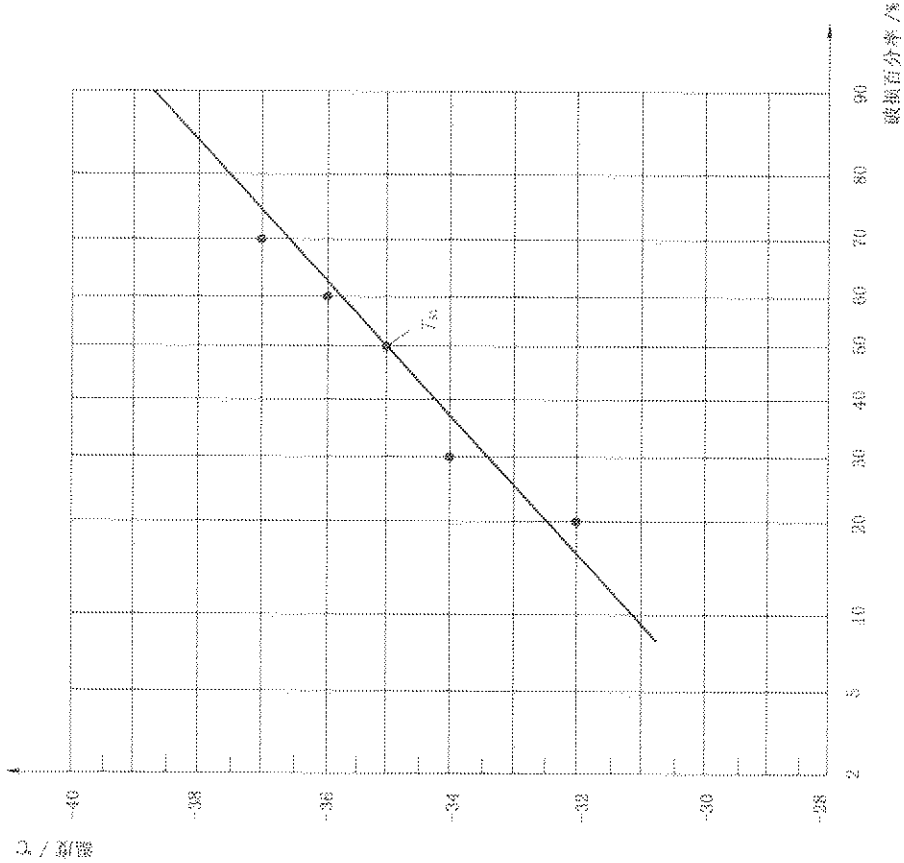
图 7 图解法测定脆化温度 T_{se} 示例
