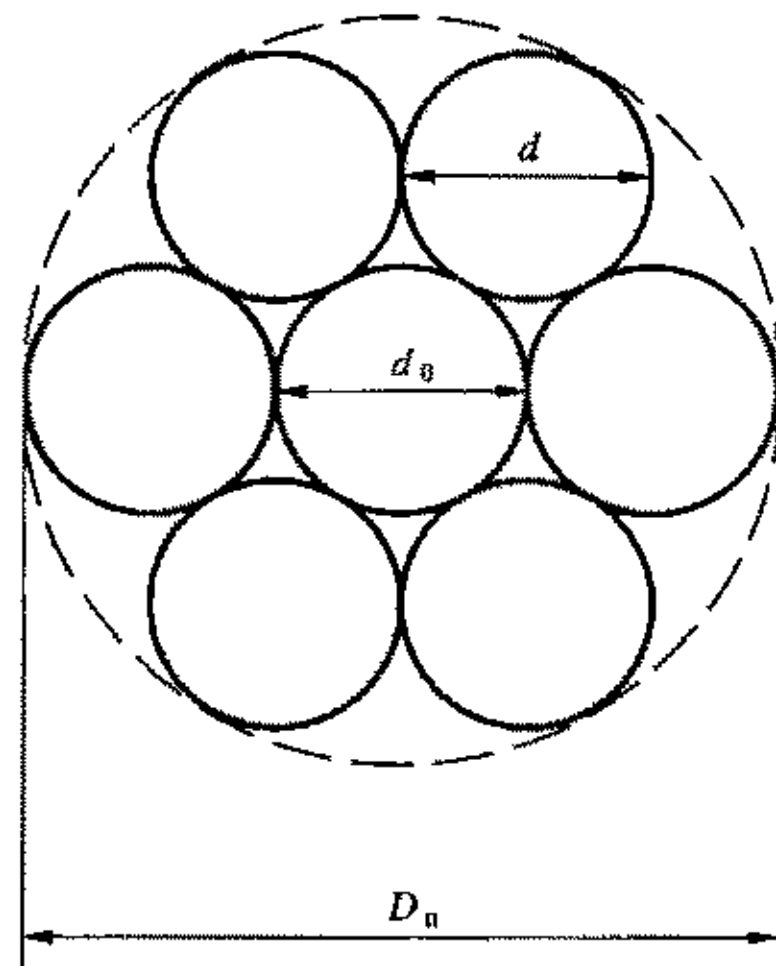
图 3 1×7 结构钢绞线外形示意图
