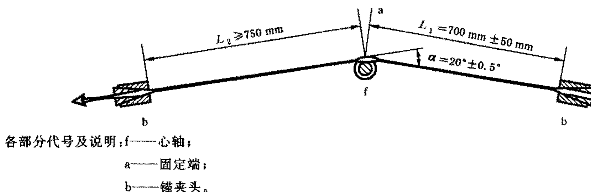
图 B.1 偏斜拉伸试验装置
