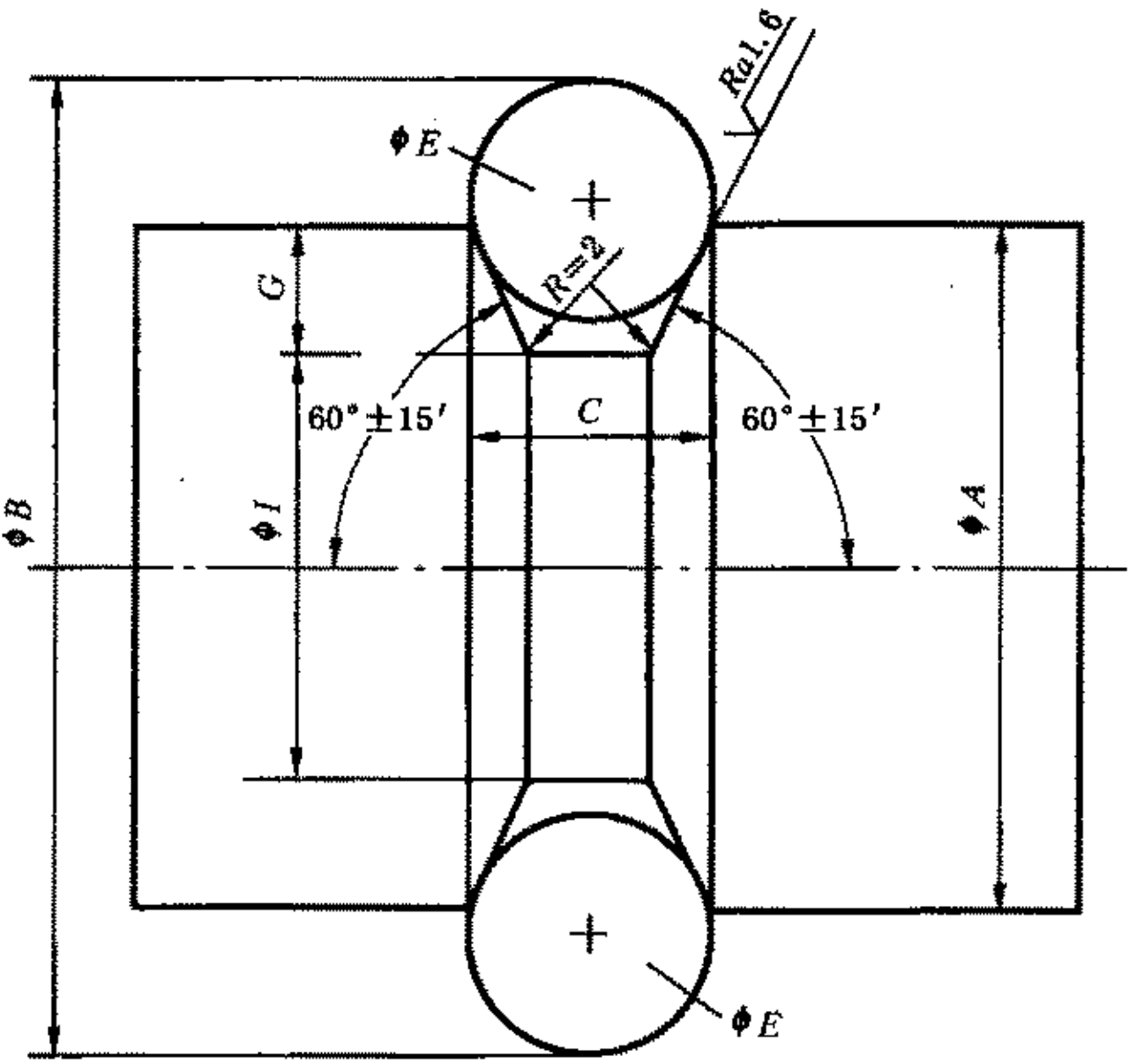
图 B.2 心轴
