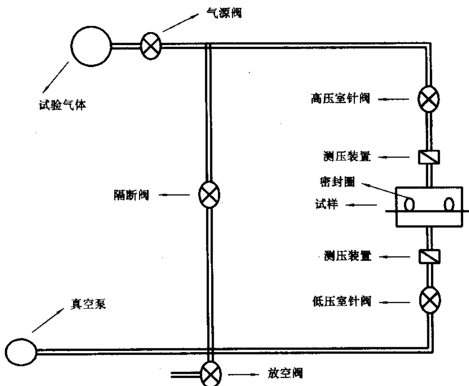
图 1 透气仪
