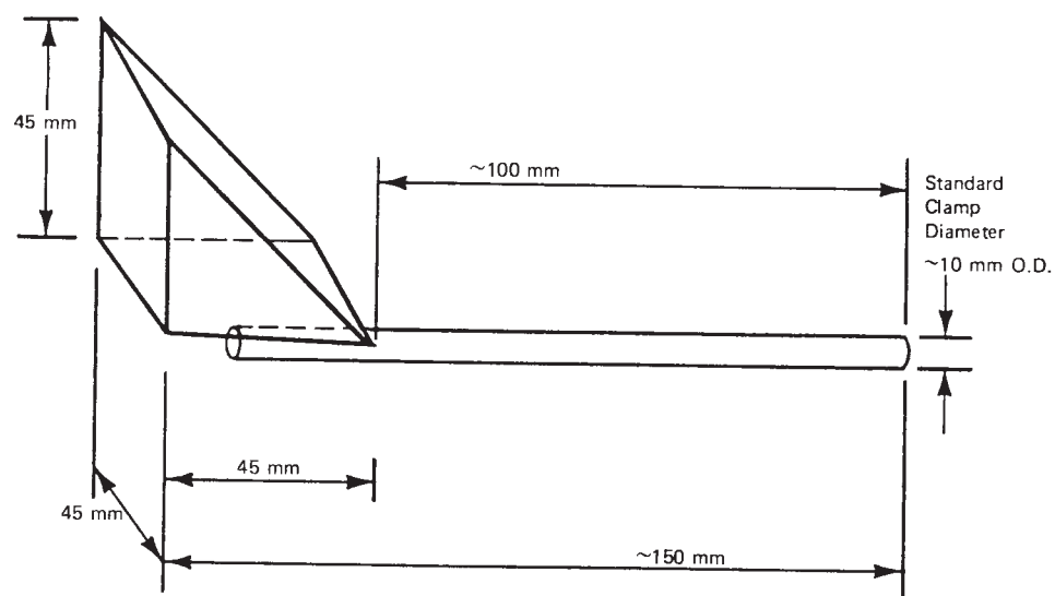
FIG. 3 Vibrator Holder
