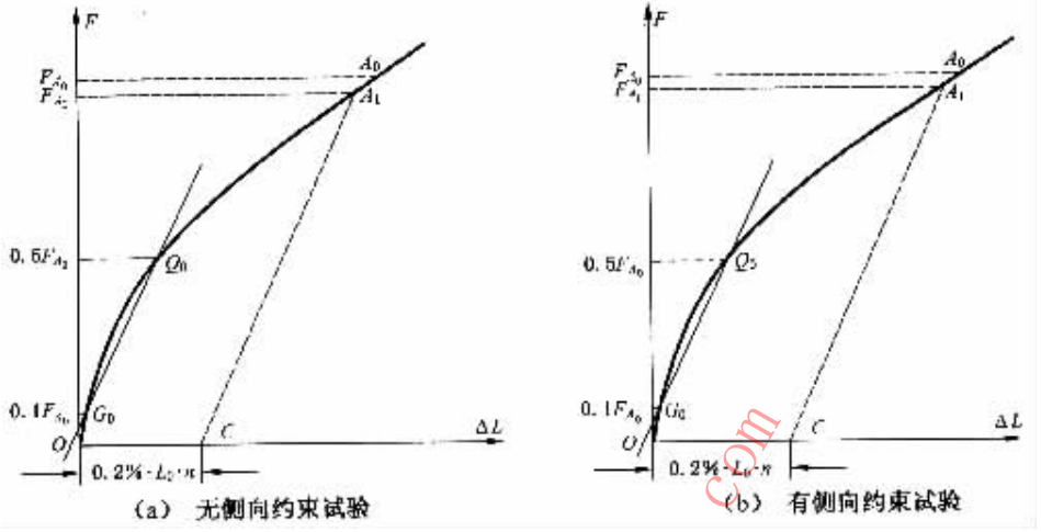
图 10 逐步逼近法求 F_{pc}
