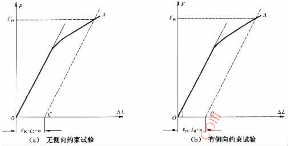
图9 图解法求 F_{pc}
