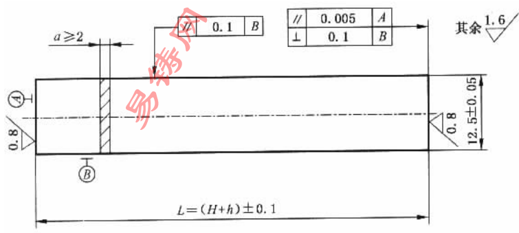
图 3 矩形板试样
