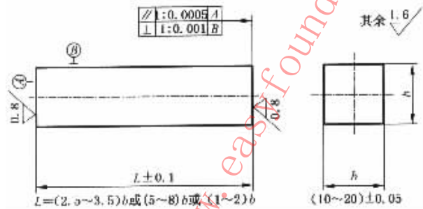
图 2 正方形柱体试样
