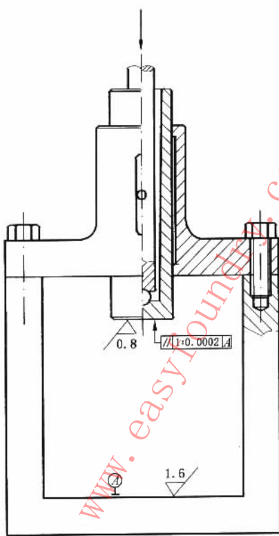
图 5 力导向装置示意图
