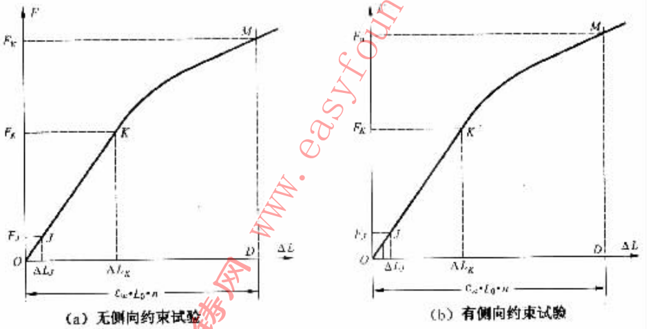
图 11 图解法求 F_{tc}
