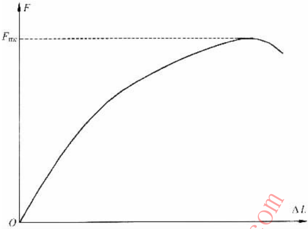
图 13 作图法求 F_{mc}
