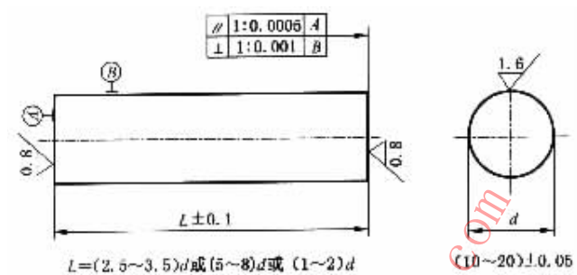
图 1 圆柱体试样
