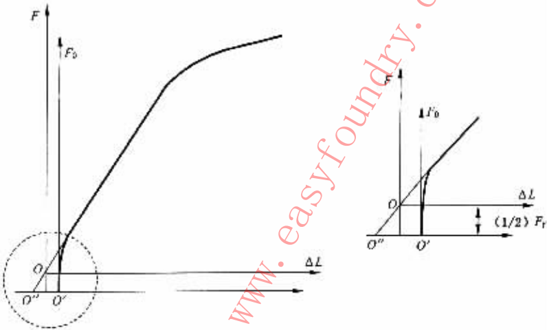
图 8 图解法确定实际压缩力 F
