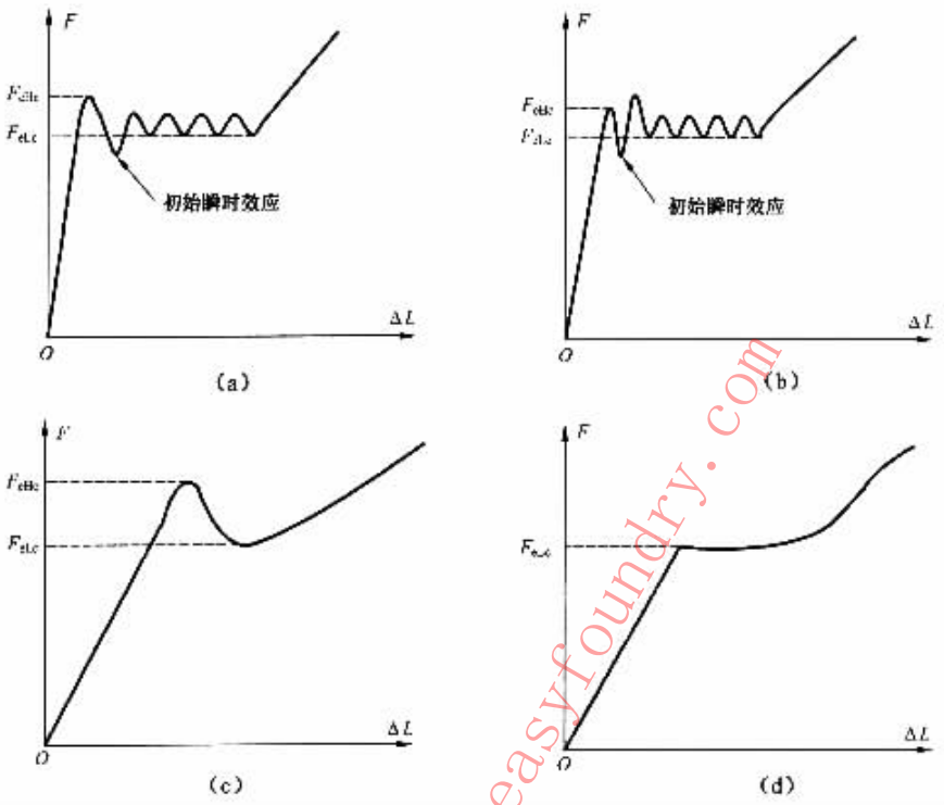
图 12 图解法求 F_{eHc} 和 F_{eLc}
