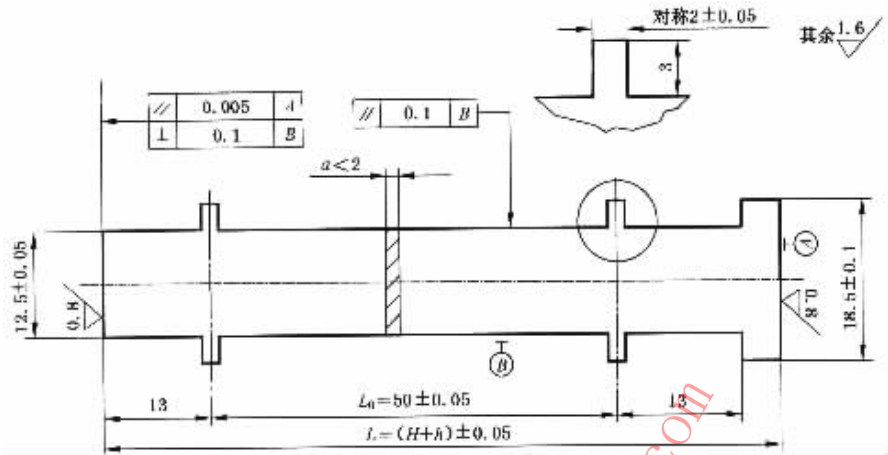
图4 带凸耳板状试样
