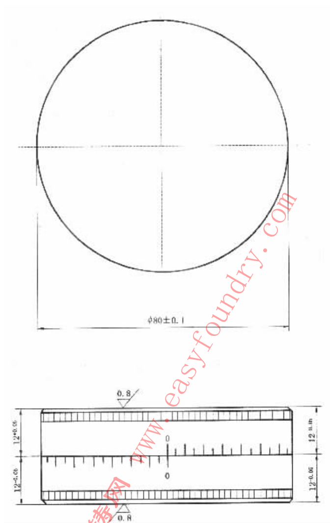
图6 调平垫块
