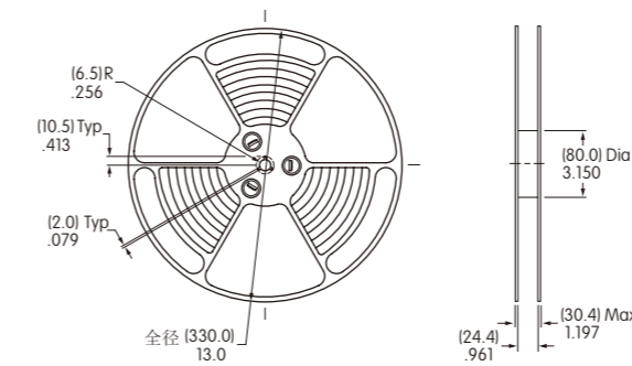
用于JSO404FP4-R 和 JSO408FP4-R的盘尺寸
