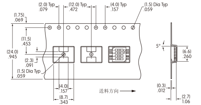
用于JSO404FP4-R的磁带尺寸
