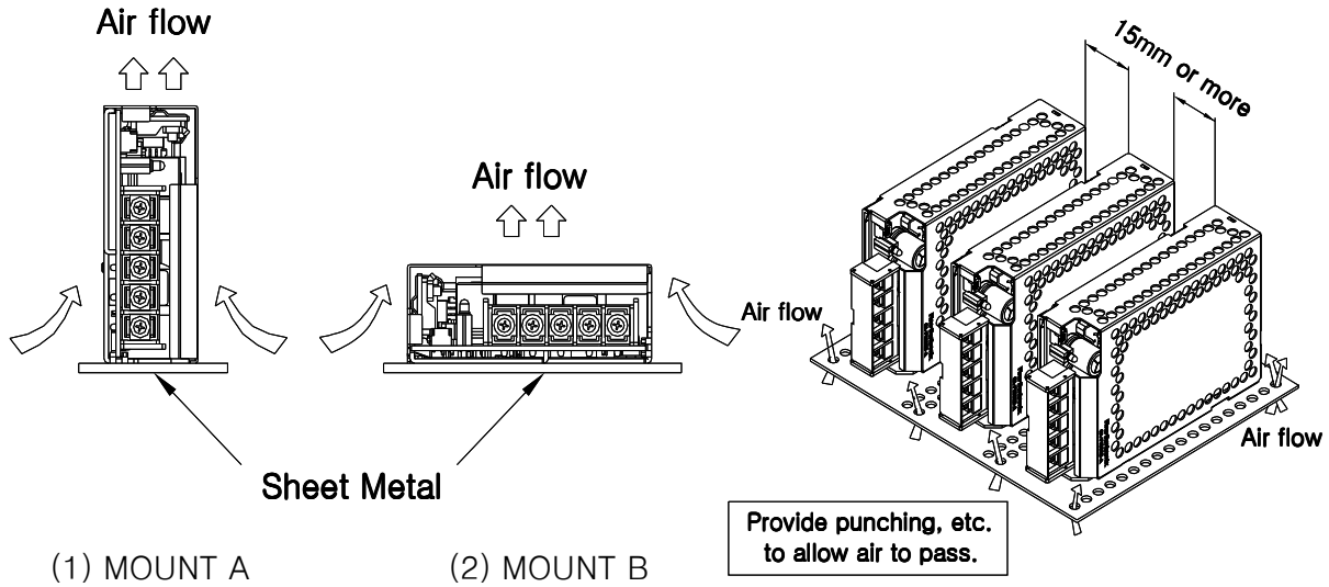
Fig 1. 기본 실장법
