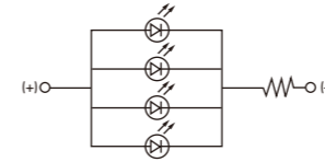
T-1 双引脚
