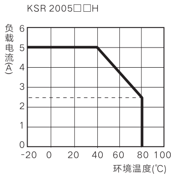
环境温度 - 负载电流
