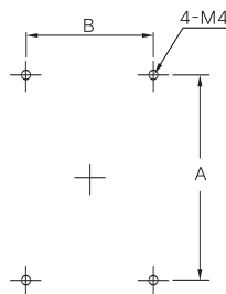
扩展型表面安装 加工尺寸图
