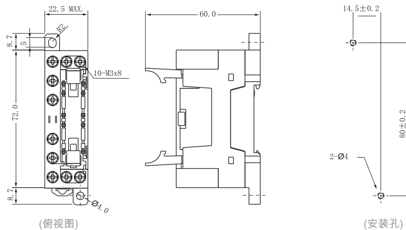
外形图
