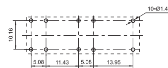
PCB 配置图(仰视图)
