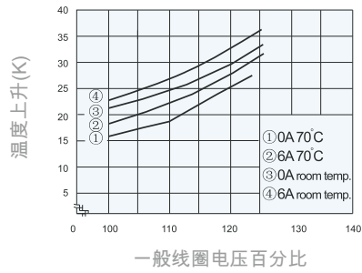
线圈温度
