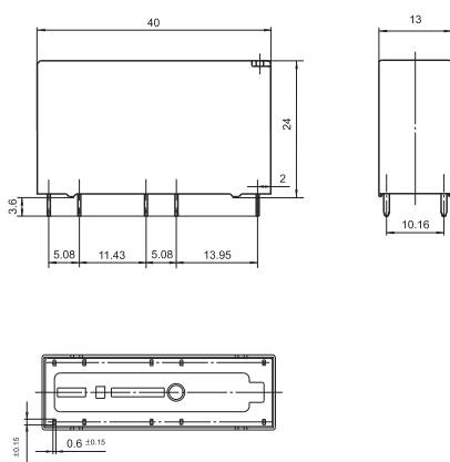
外形图(单位:毫米)
