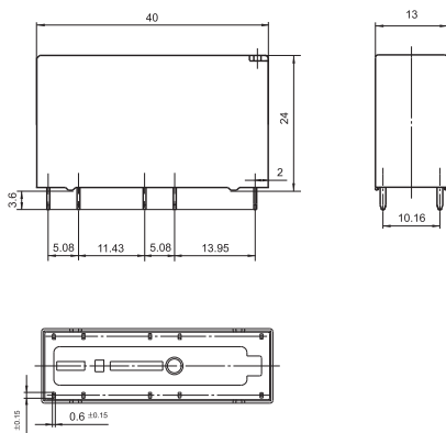
外形图(单位:毫米)
