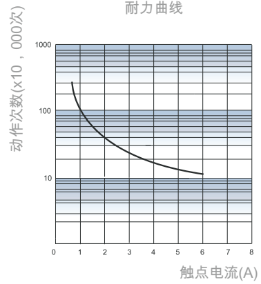
耐力曲线
