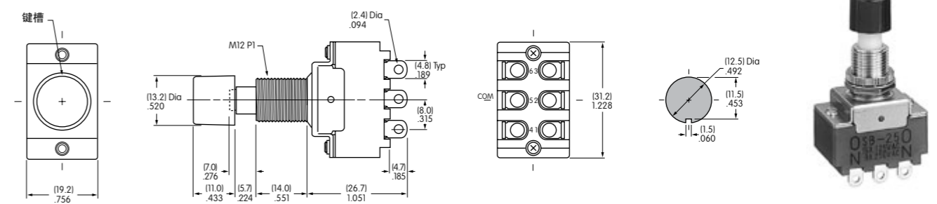
面板厚度 .193" (4.9mm) 与AT414黑色盖帽一起提供
