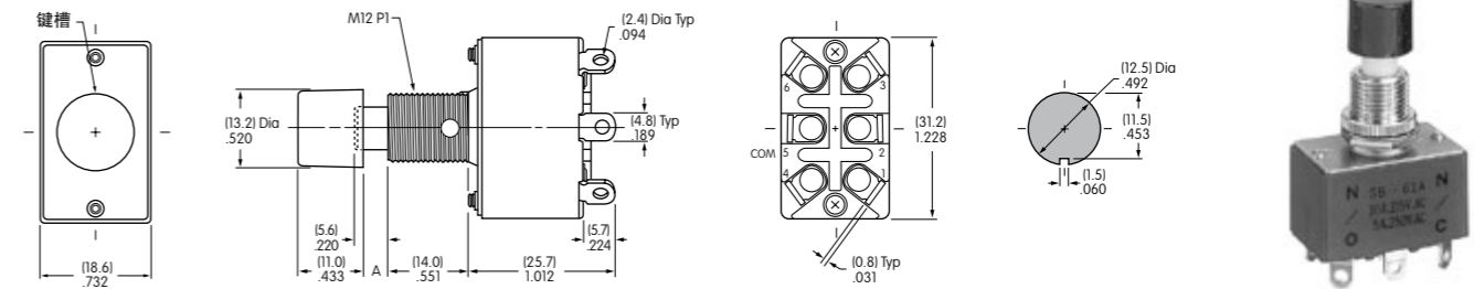
尺寸A: .169" (4.3mm)对于SB61型号和 .130" (3.3mm) 对于SB63型号。 面板厚度 .193" (4.9mm) 与AT414黑色盖帽一起提供
