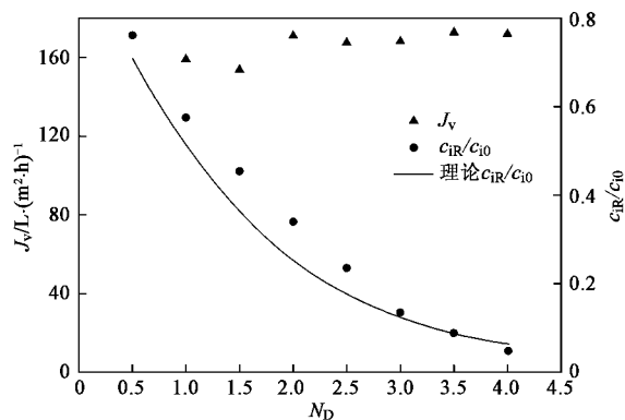
图 7 超滤杯中 \text{Pb}^{2+} 的相对浓度和膜通量随全过滤倍数的变化
