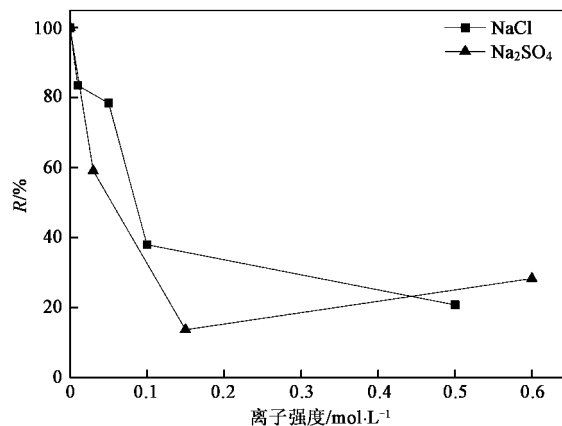
图 4 离子强度对 Pb^{2+} 截留率的影响
