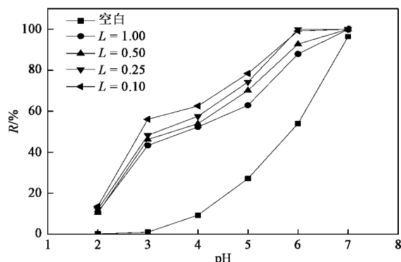
图 2 在不同的壳聚糖添加量下,pH 值对 Pb^{2+} 截留率的影响 Fig. 2 Effect of pH on lead removal at different Pb^{2+} /chitosan ratios
