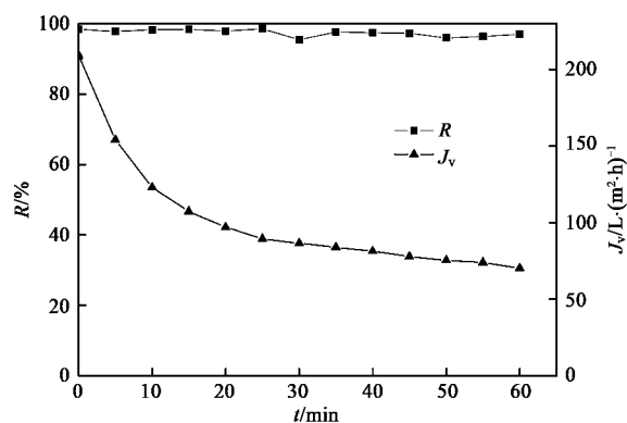
图 6 浓缩时间对膜通量及 \text{Pb}^{2+} 截留率的影响
