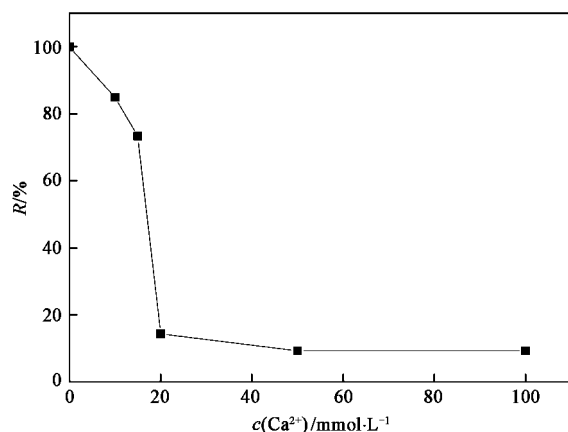
图 5 \text{Ca}^{2+} 浓度对 \text{Pb}^{2+} 截留率的影响
