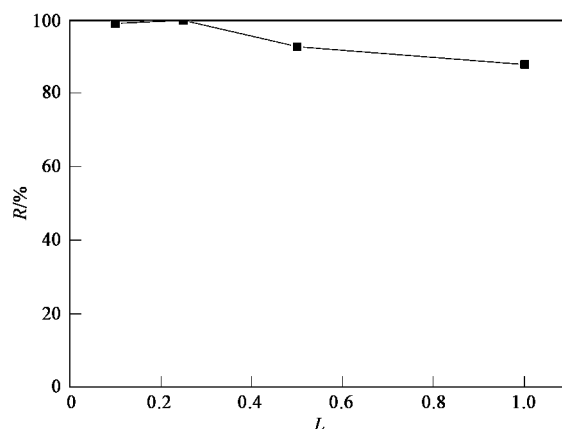
图 3 pH = 6.0 时 Pb^{2+} /壳聚糖装载量比 L 对 Pb^{2+} 截留率的影响
