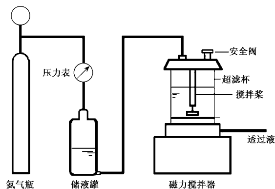
图1 超滤实验流程示意
